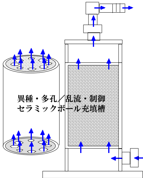
標準機器の分解構造図
